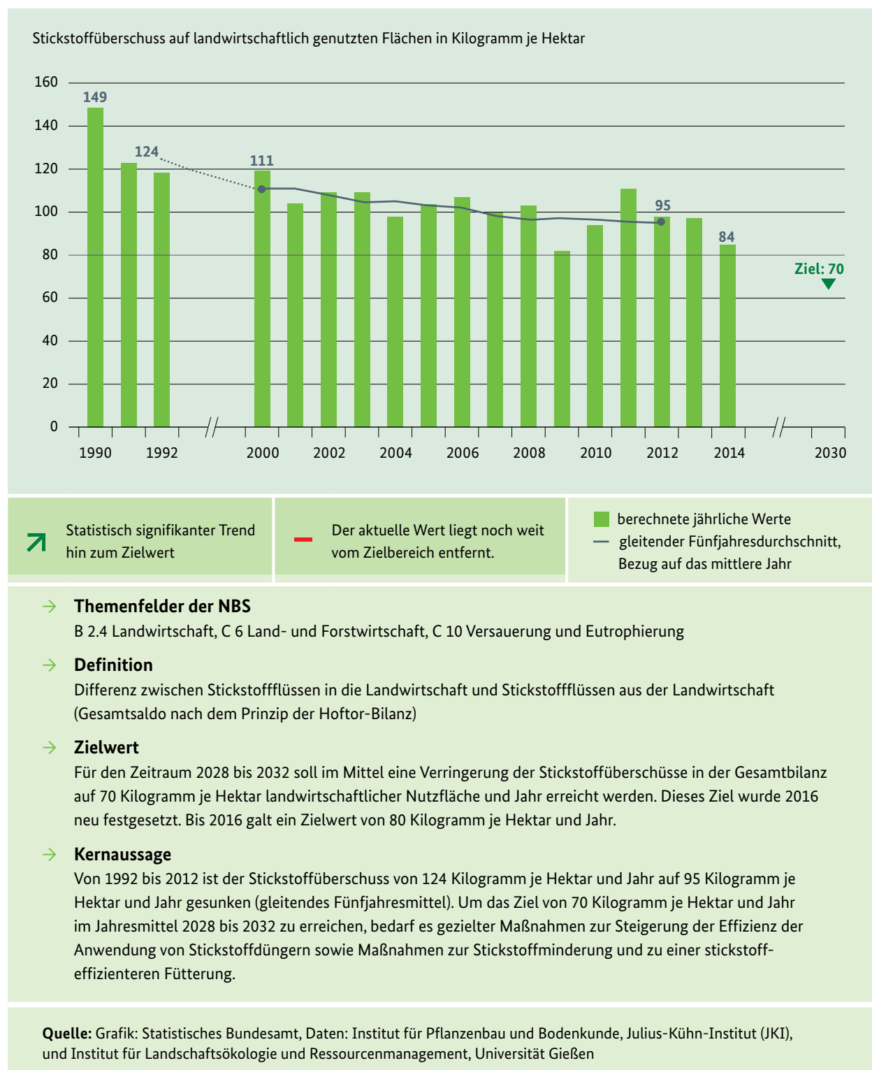
Abbildung 16: Stickstoffüberschuss der Landwirtschaft
